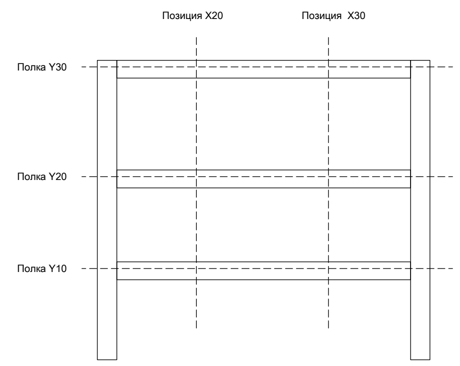
Адресация ячеек Вид на стеллаж со стороны крана-штабелера
