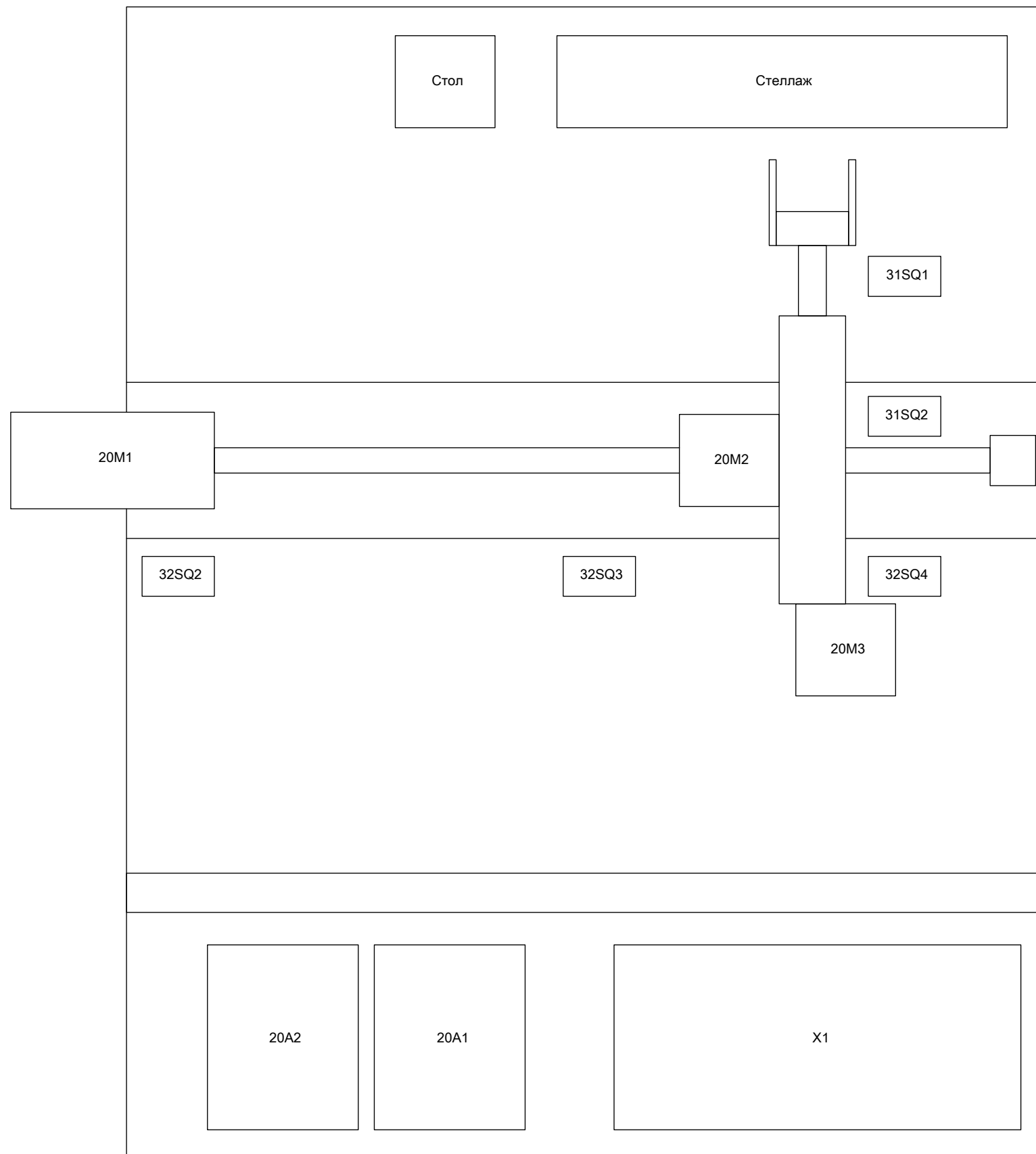
Вид сверху
