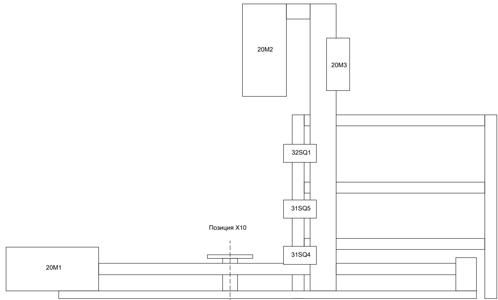
Вид на стеллаж со стороны крана-штабелера
